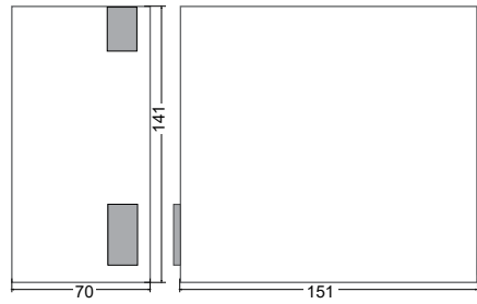
机械尺寸
